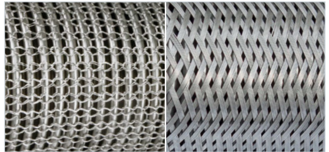
Weich gegen weich! (Drahtgestrick/Drahtgeflecht) Soft for soft! (knit wire mesh/wire mesh)
